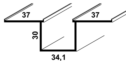
Hutprofil KLE 30/25/35/6 N Nr. S 2036 - 756
